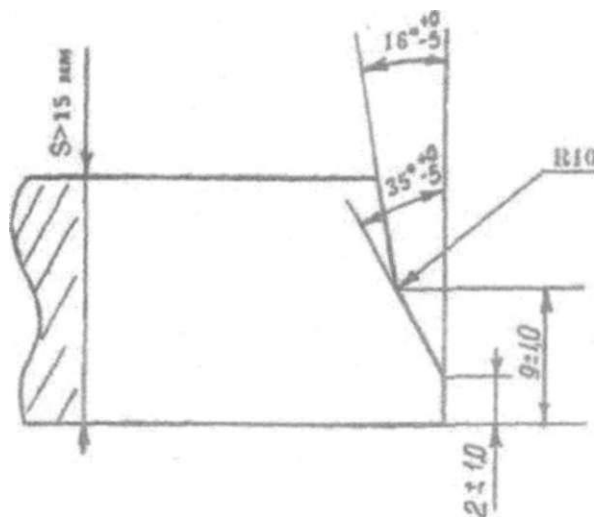
Рис 1 Разделка кромок торцов трубы.
